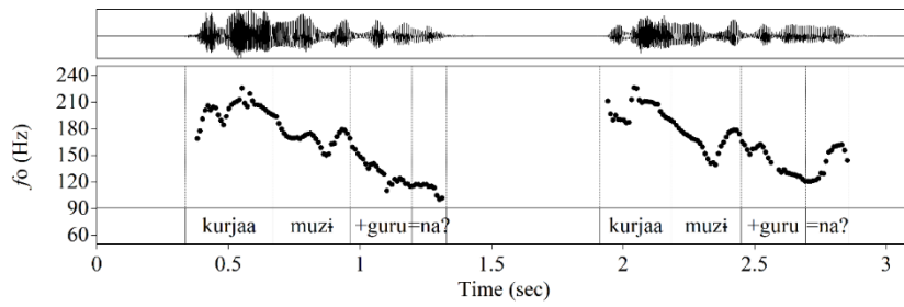
図 1 上昇句末音調を欠く YNQ (左) とそれを伴う YNQ (右) (3a) の音声波形と f_0 曲線
