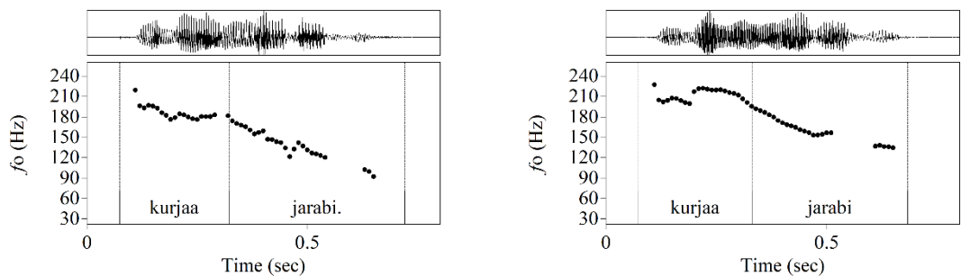
図 6 平叙文 (6b) (左) と文末疑問標識を伴わない YNQ (6c) (右) の音声波形と f_0 曲線
