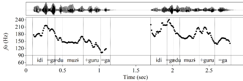
図 2 上昇句末音調を欠く WHQ (左) とそれを伴う WHQ (右) (3b) 音声波形と f_0 曲線
