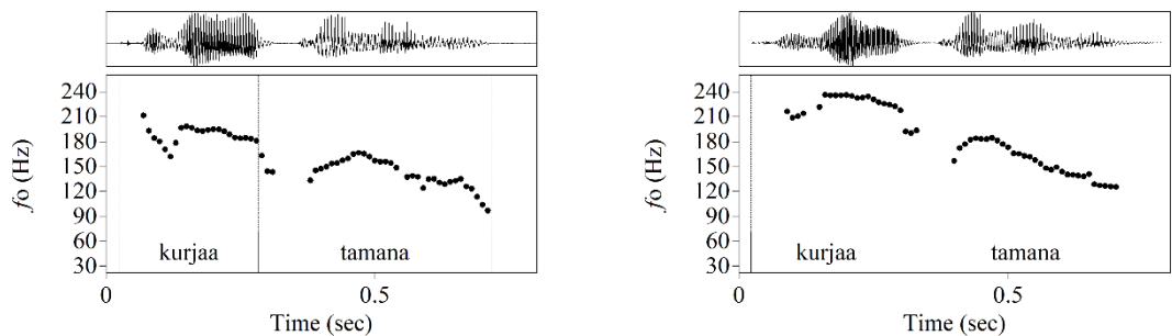
図 5 平叙文 (6a) (左) と文末疑問標識を伴わない YNQ (6b) (右) の音声波形と f_0 曲線
