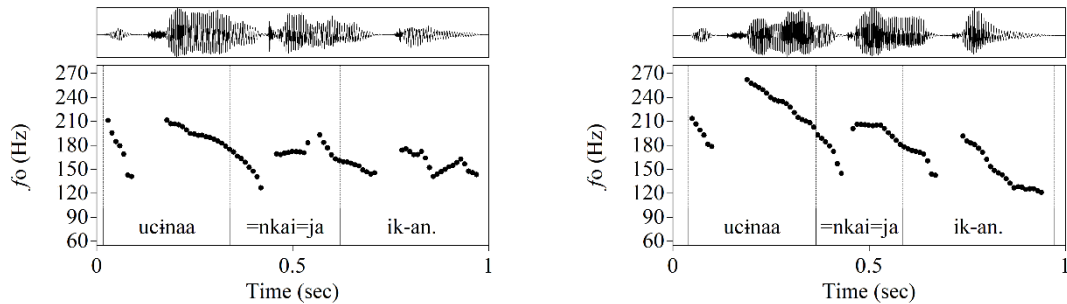
図 4 平叙文 (5a) (左) と文末疑問標識を伴わない YNQ (5b) (右) の音声波形と f_0 曲線
