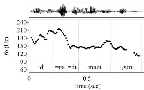
図 3 文末疑問標識を欠く WHQ (4) 音声波形と f_0 曲線
